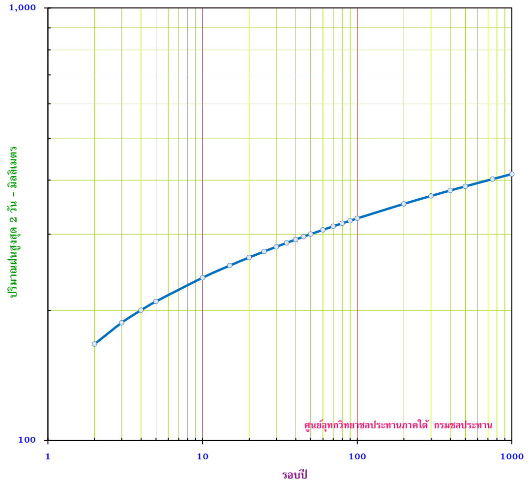
กราฟแสดง ปริมาณฝนสูงสุด 2 วัน ขนาดรอบปีต่างๆ สถานี 430091 เขื่อนบางวาด ชป.ภูเก็ต อ.กะทู้ จ.ภูเก็ต
