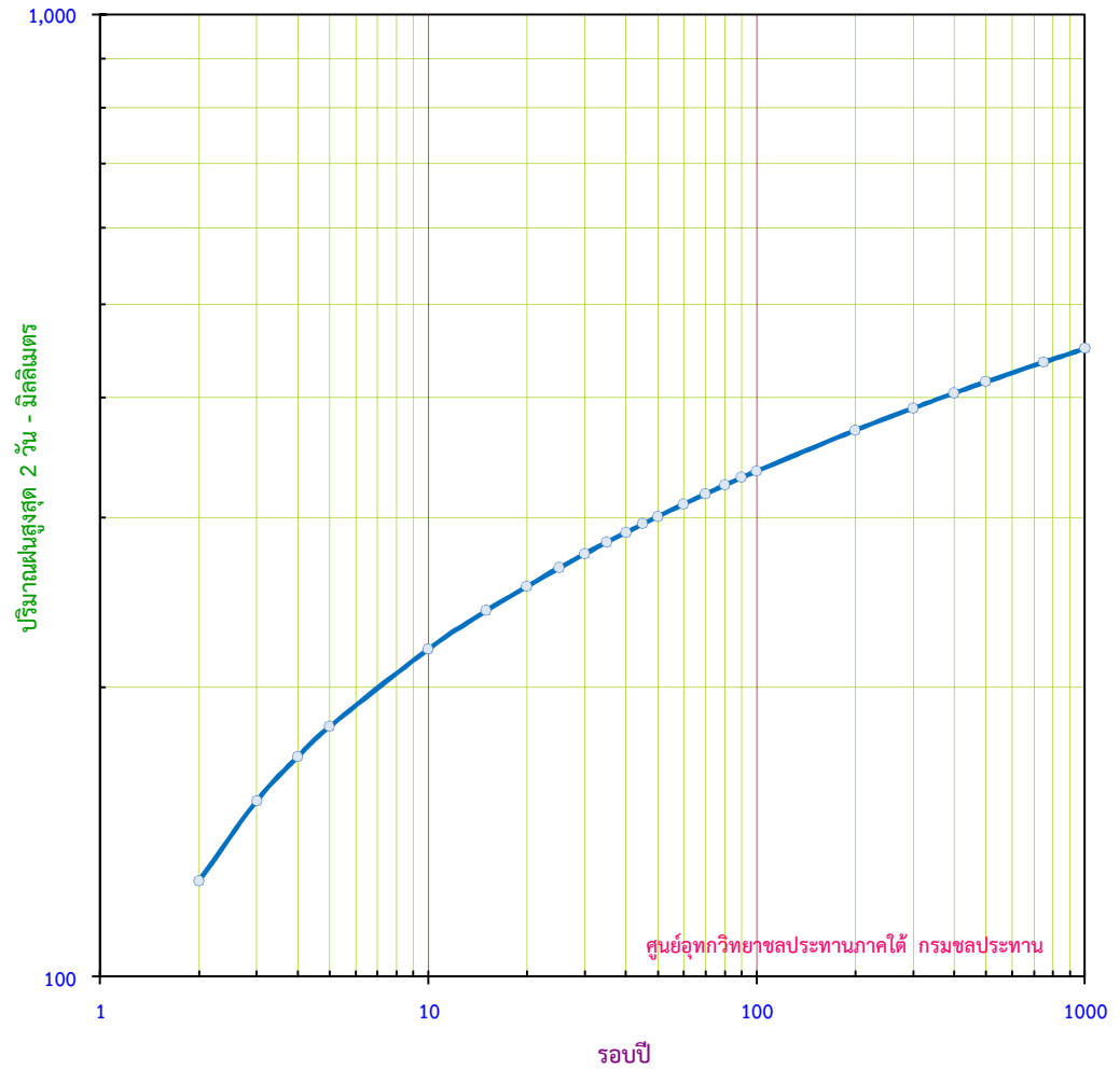
กราฟแสดง ปริมาณฝนสูงสุด 2 วัน ขนาดรอบปีต่างๆ สถานี 580221(X.113) บ.ทุ่งปราบ อ.เสตะ จ.สงขลา
