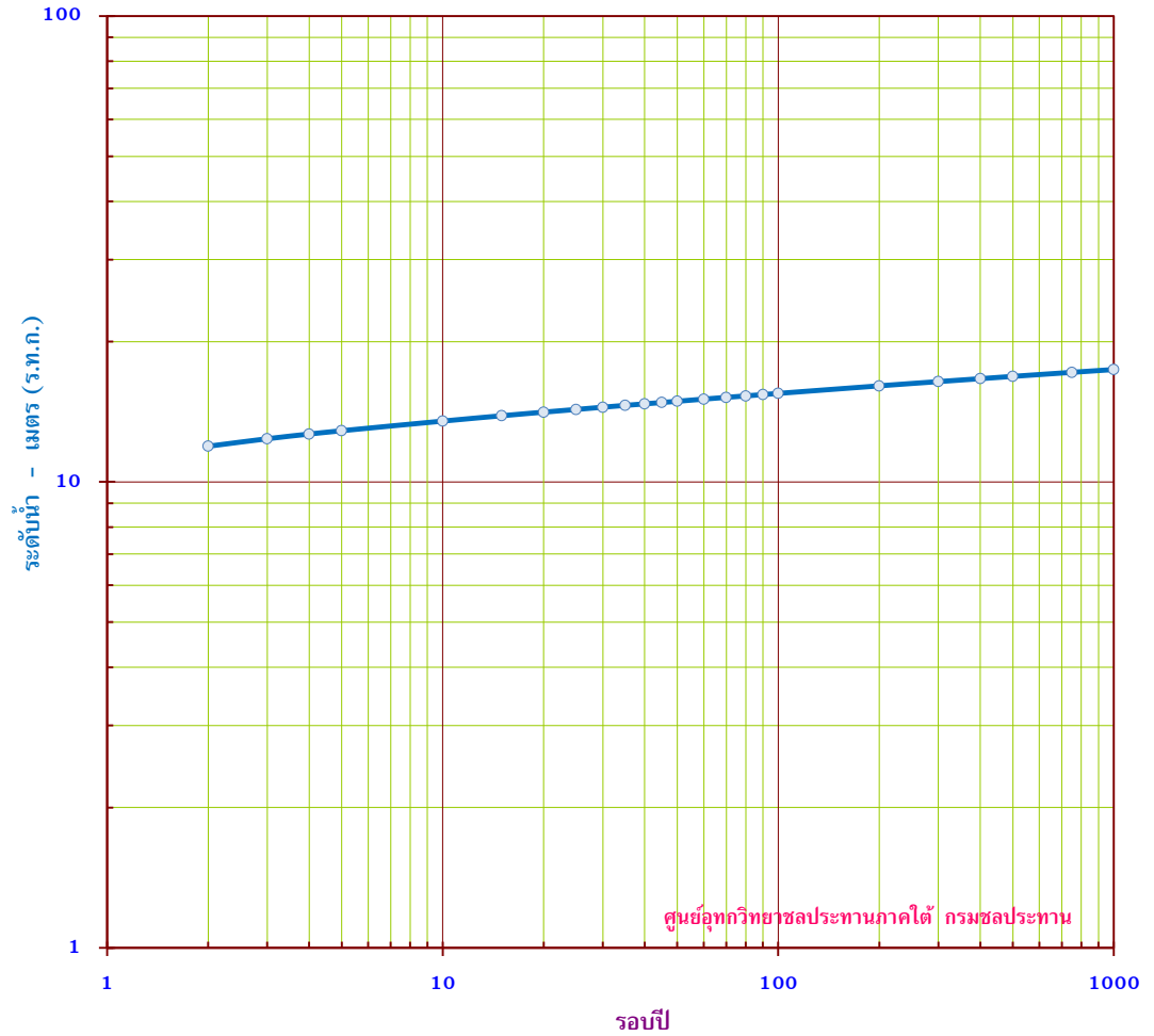
กราฟแสดง ระดับน้ำสูงสุดรายปี ขนาดรอบปีต่าง ๆ สถานี X.150 บ.วังพระเคียน อ.ละงู จ.สตูล
