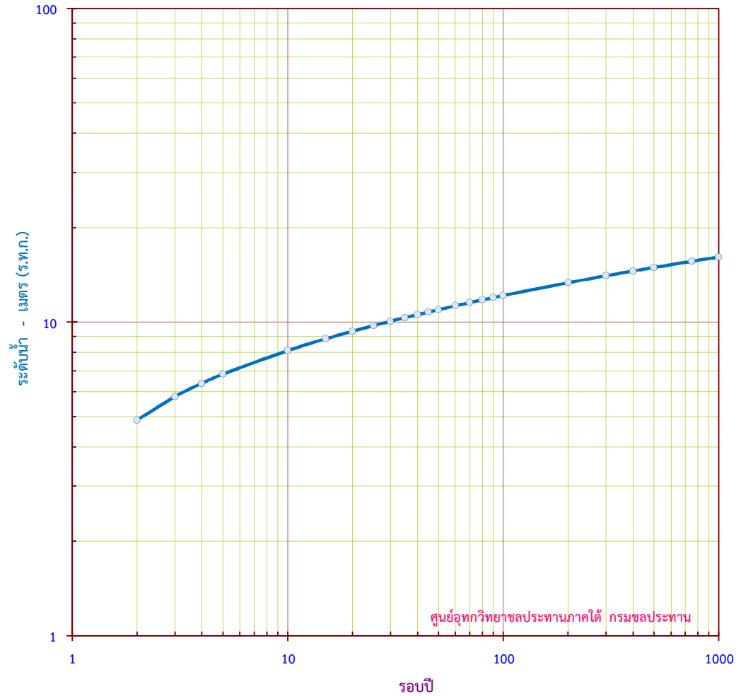
กราฟแสดง ระดับน้ำสูงสุดรายปี ขนาดรอบปีต่างๆ สถานี X.44 บ.หาดใหญ่ใน อ.หาดใหญ่ จ.สงขลา
