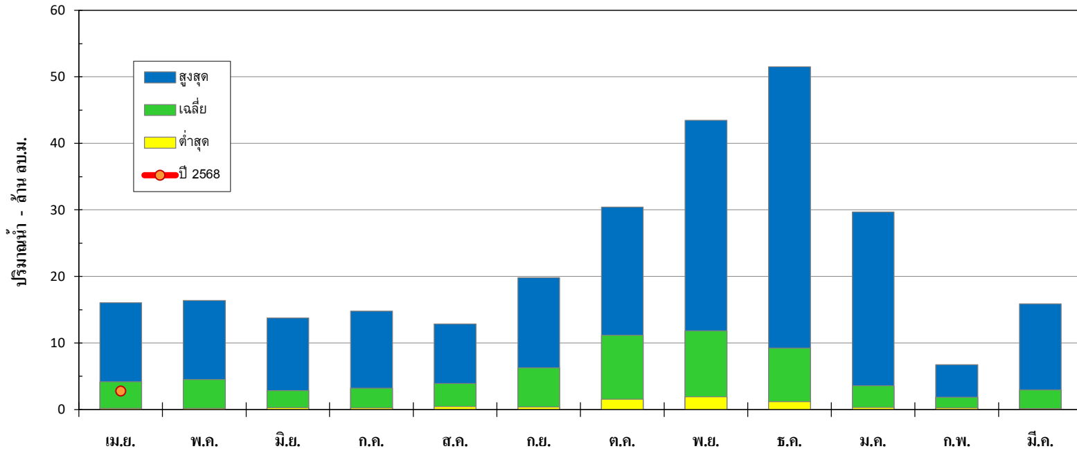
กราฟปริมาณน้ำท่ารายเดือน คลองห้ำป้ง ปีน้ำ 2522-2566 สถานี X.113 บ.ทุ่งปราบ อ.เสเดา จ.สงขลา
