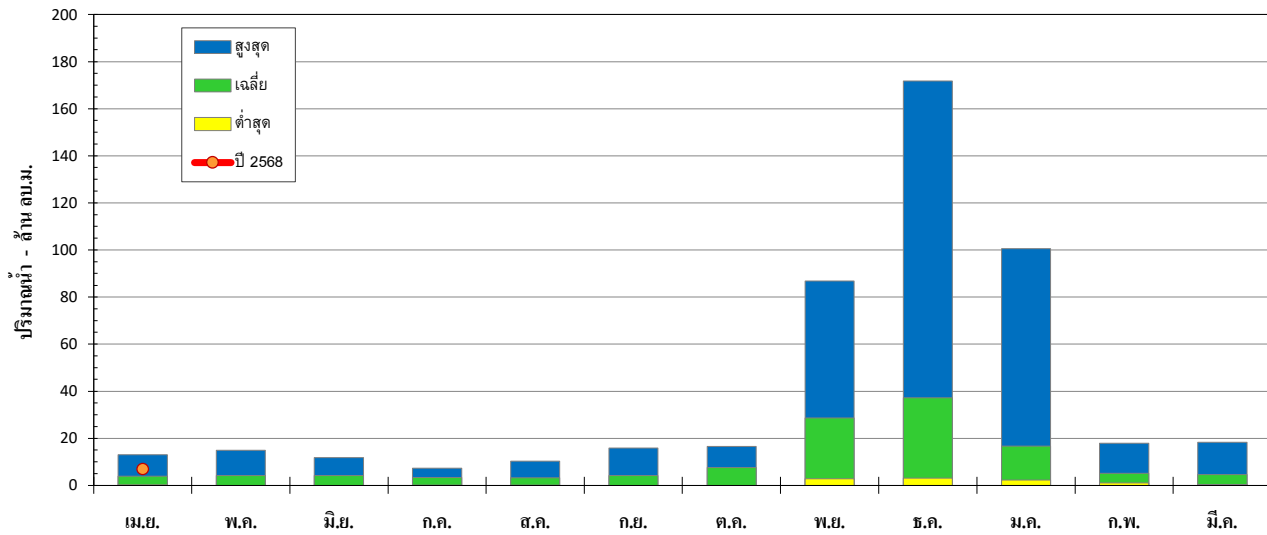
กราฟปริมาณน้ำท่ารายเดือน คลองหะ ปีน้า 2534-2566 สถานี X.174 บ.คลองหะ อ.หาดใหญ่ จ.สงขลา
