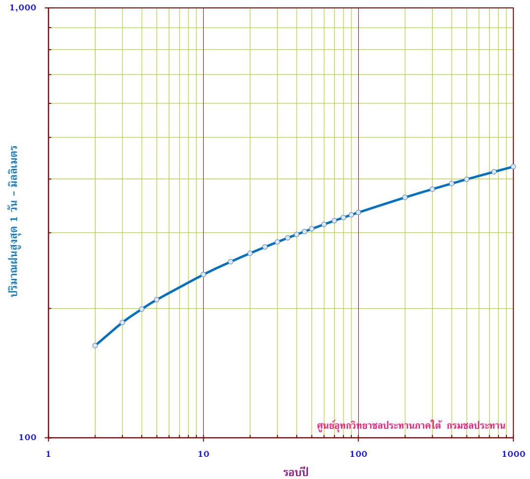
กราฟแสดง ปริมาณฝนสูงสุด 1 วัน ขนาดรอบปีต่างๆ สถานี 340231(X.187) บ.หินदान อ.ตะกั่วป่า จ.พังงา
