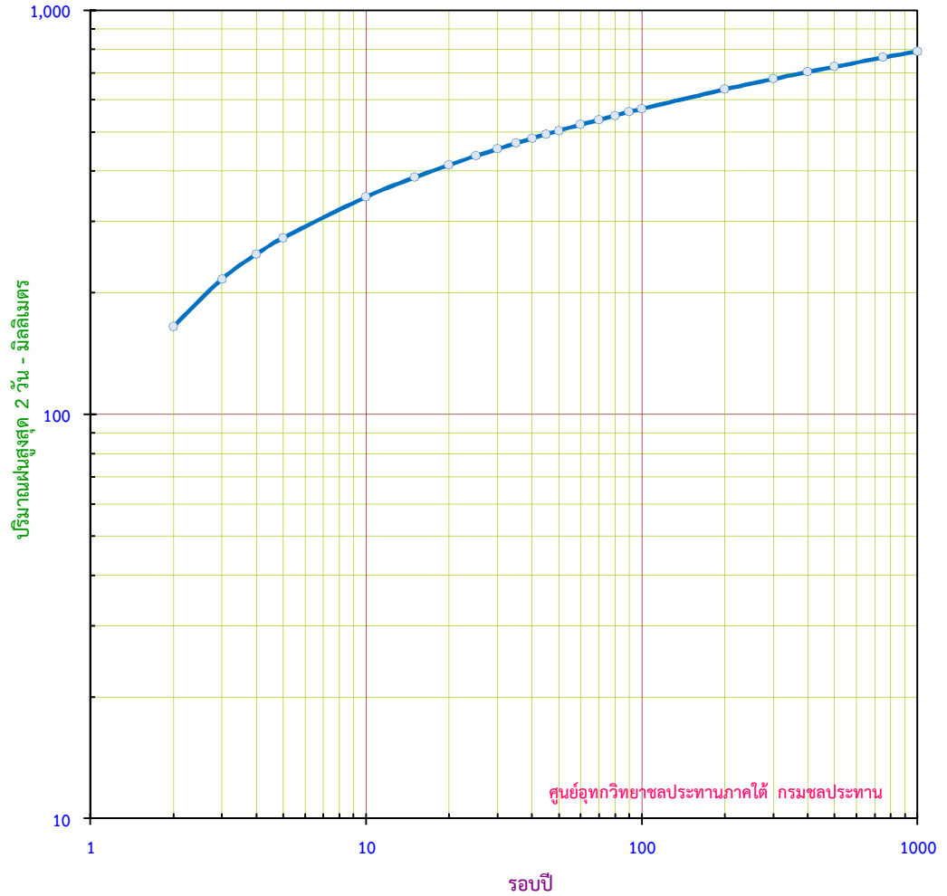
กราฟแสดง ปริมาณฝนสูงสุด 2 วัน ขนาดรอบปีต่างๆ สถานี 580411 บ.นาทองสุข อ.นาทม่อม จ.สงขลา
