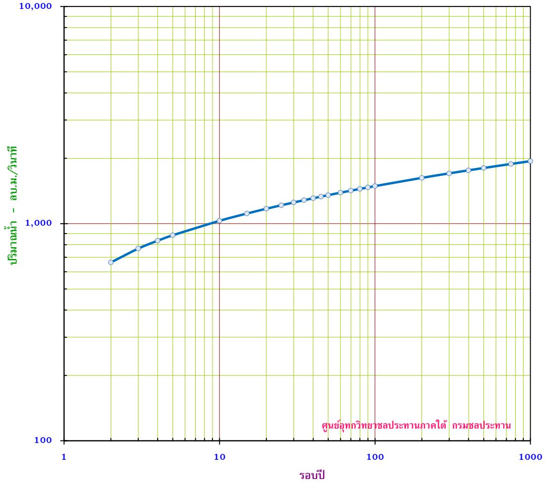
กราฟแสดง ปริมาณน้ำสูงสุดรายปี ขนาดรอบปีต่างๆ สถานี X.187 บ.หินदान อ.ตะกั่วป่า จ.พังงา
