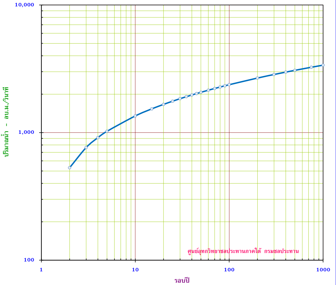
กราฟแสดง ปริมาณน้ำสูงสุดรายปี ขนาดรอบปีต่างๆ สถานี X.228 บ.กลาง อ.เมือง จ.ตรัง
