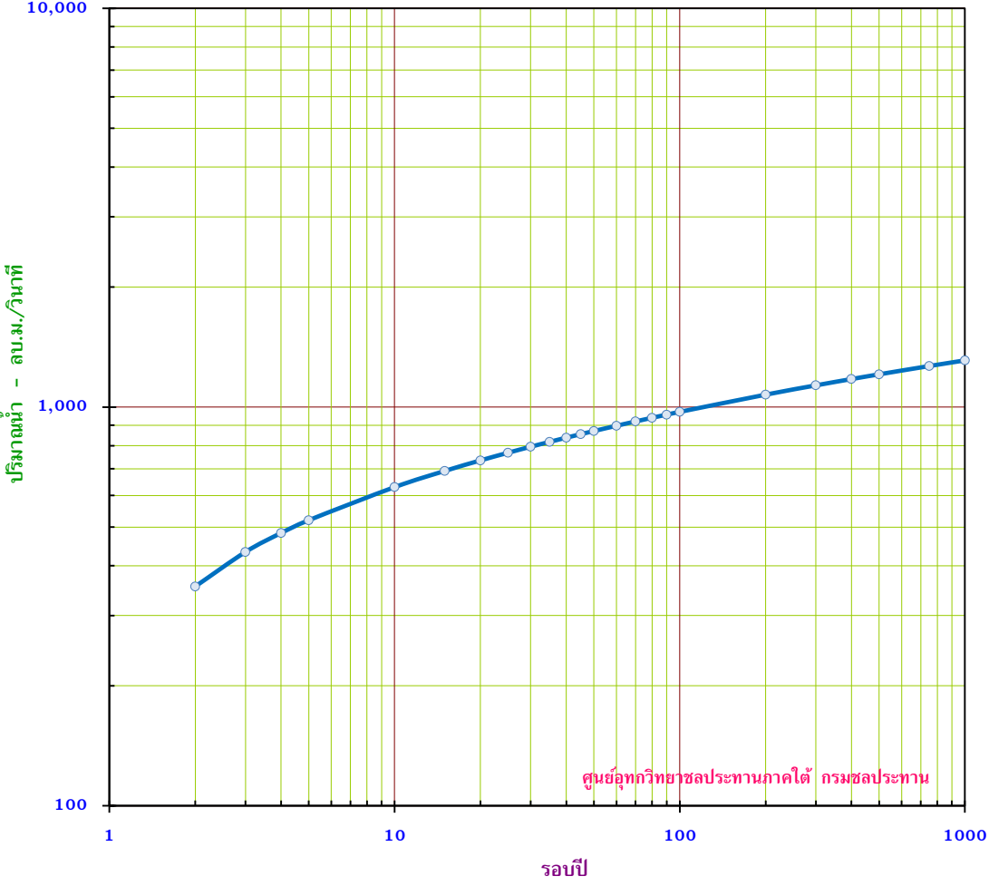
กราฟแสดง ปริมาณน้ำสูงสุดรายปี ขนาดรอบปีต่างๆ สถานี X.234 บ.ป่าหมาก อ.เมือง จ.ตรัง
