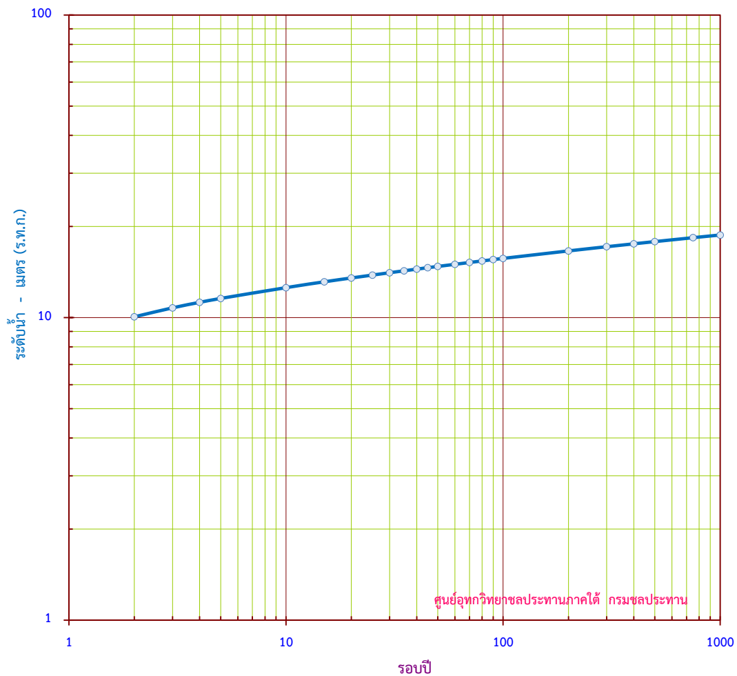
กราฟแสดง ระดับน้ำสูงสุดรายปี ขนาดรอบปีต่างๆ สถานี X.158 บ.วังครก อ.ท่าแซะ จ.ชุมพร
