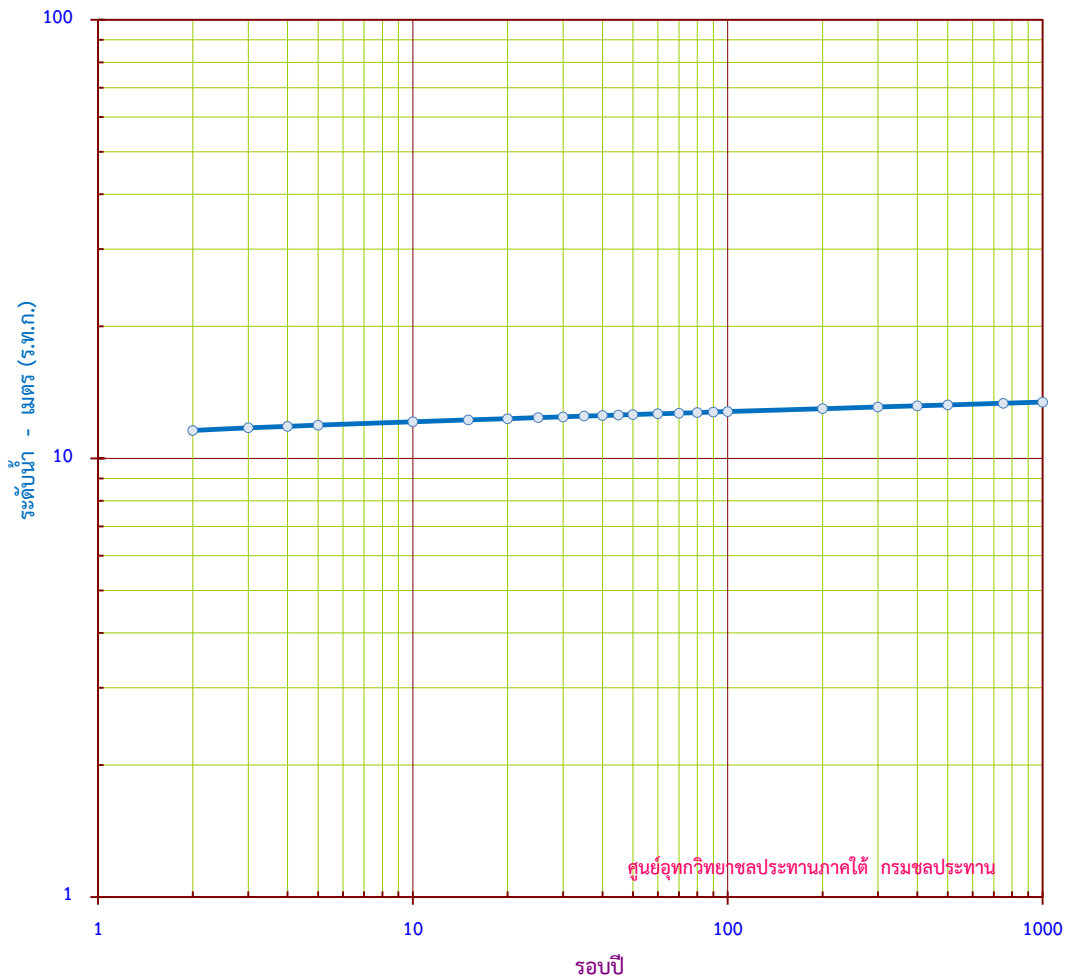
กราฟแสดง ระดับน้ำสูงสุดรายปี ขนาดรอบปีต่างๆ สถานี X.167 บ.เสาชาง อ.ร่อนพิบูลย์ จ.นครศรีธรรมราช
