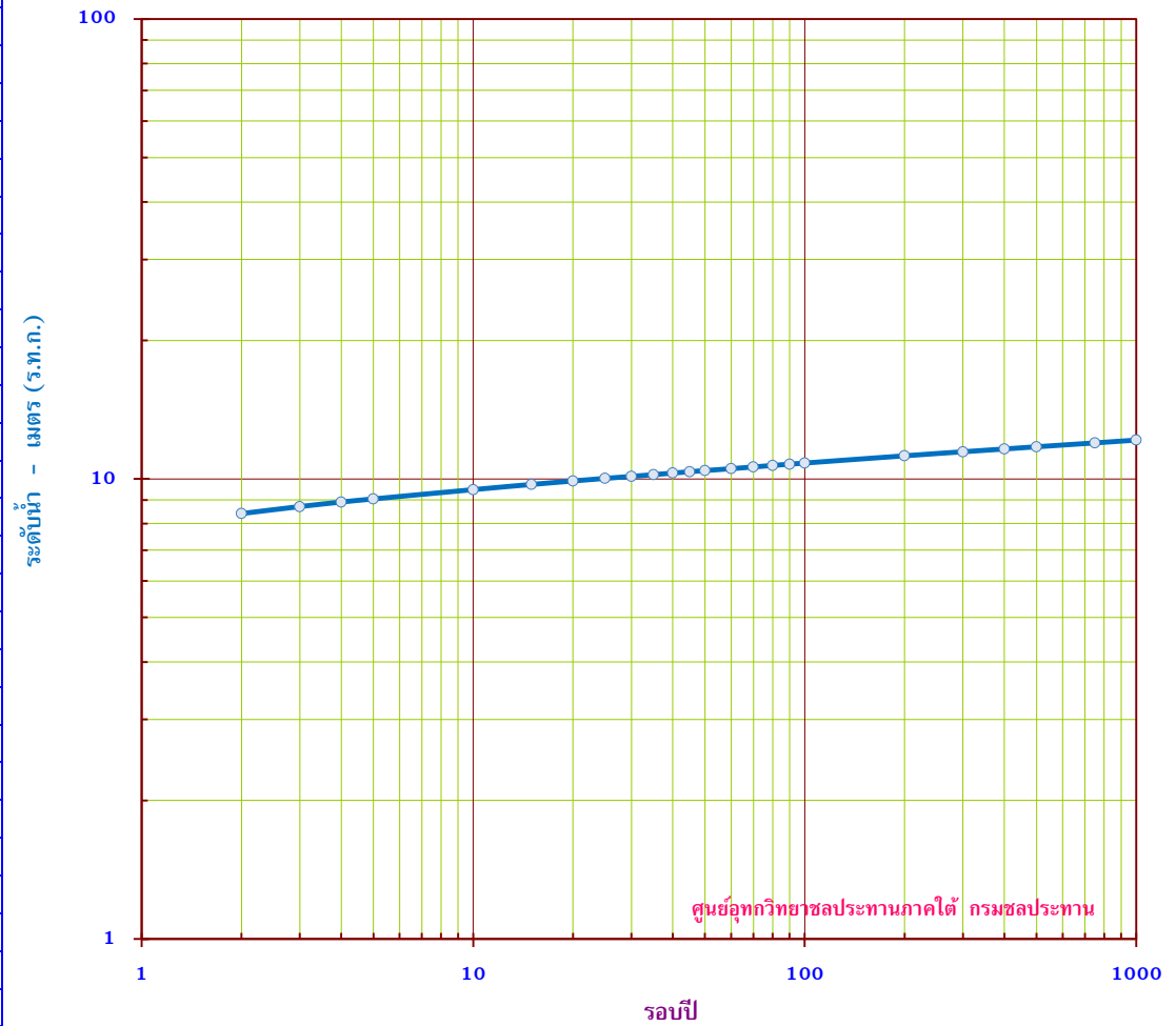
กราฟแสดง ระดับน้ำสูงสุดรายปี ขนาดรอบปีต่าง ๆ สถานี X.187 บ.หินदान อ.ตะกั่วป่า จ.พังงา
