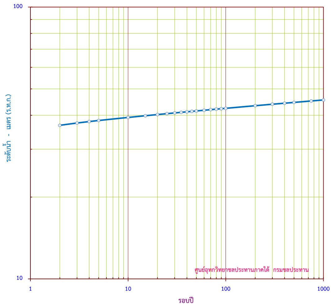
กราฟแสดง ระดับน้ำสูงสุดรายปี ขนาดรอบปีต่างๆ สถานี X.195 บ.ต้นโพธิ์ อ.ฉวาง จ.นครศรีธรรมราช
