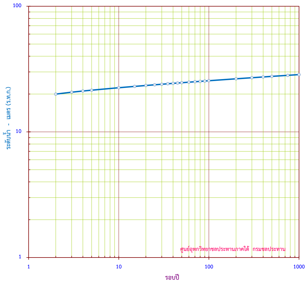
กราฟแสดง ระดับน้ำสูงสุดรายปี ขนาดรอบปีต่างๆ สถานี X.70 บ.วังก้อง อ.เมือง จ.นครศรีธรรมราช
