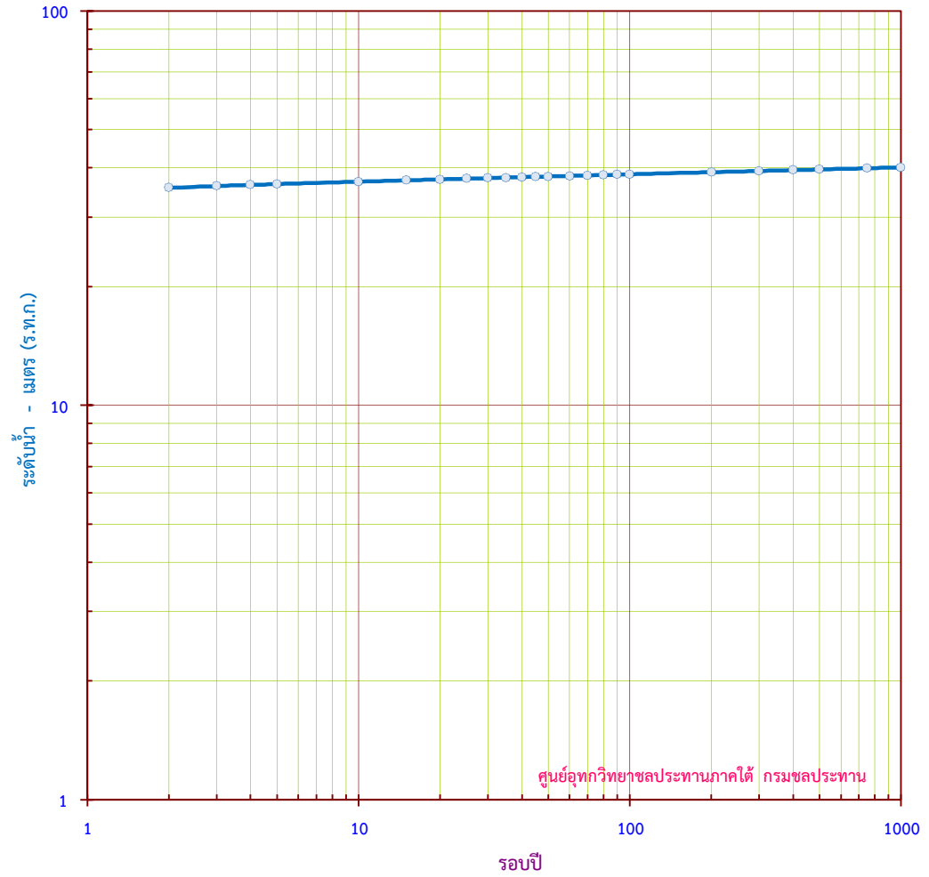
กราฟแสดง ระดับน้ำสูงสุดรายปี ขนาดรอบปีต่างๆ สถานี X.113 บ.ทุ่งปราบ อ.สะเดา จ.สงขลา
