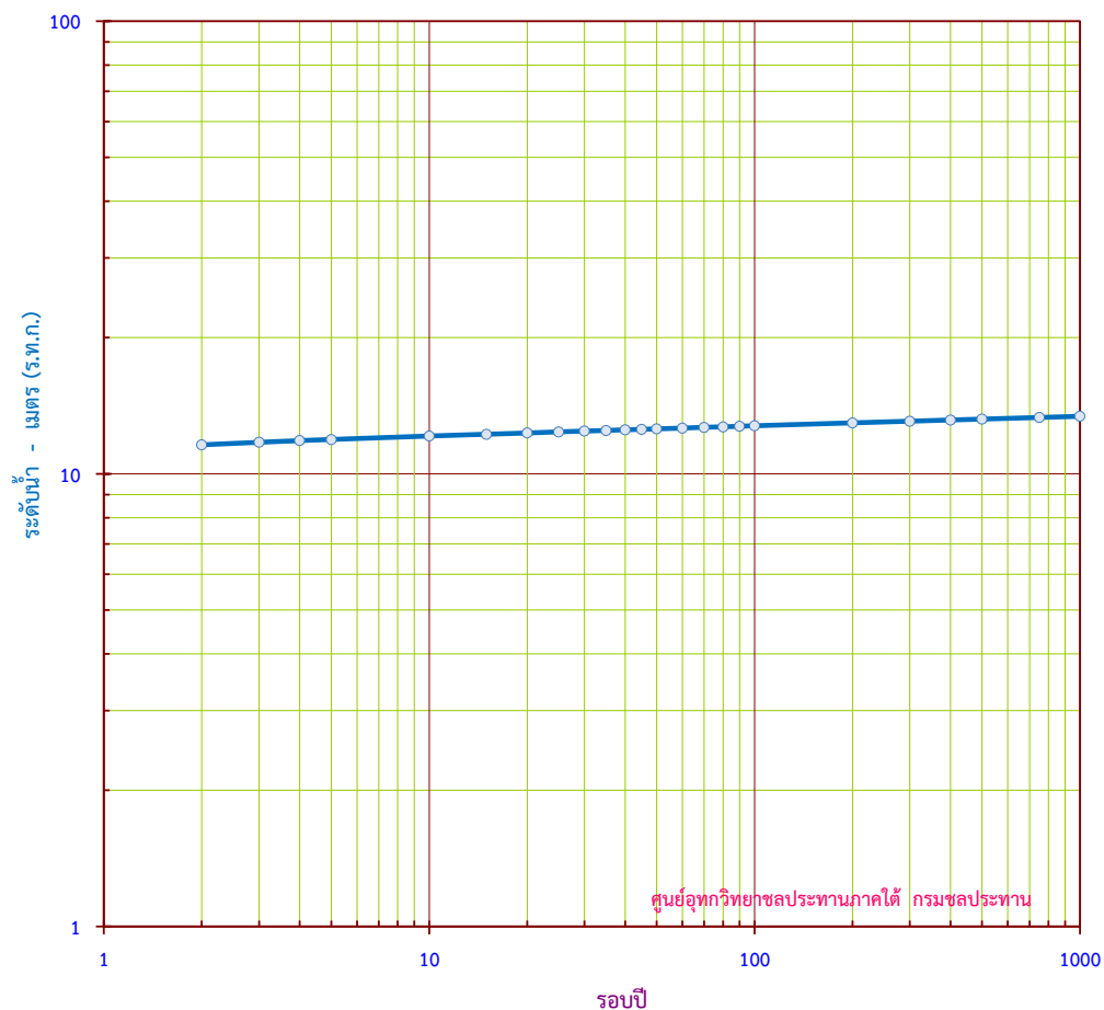
กราฟแสดง ระดับน้ำสูงสุดรายปี ขนาดรอบปีต่างๆ สถานี X.167 บ.เสาชัง อ.ร่อนพิบูลย์ จ.นครศรีธรรมราช
