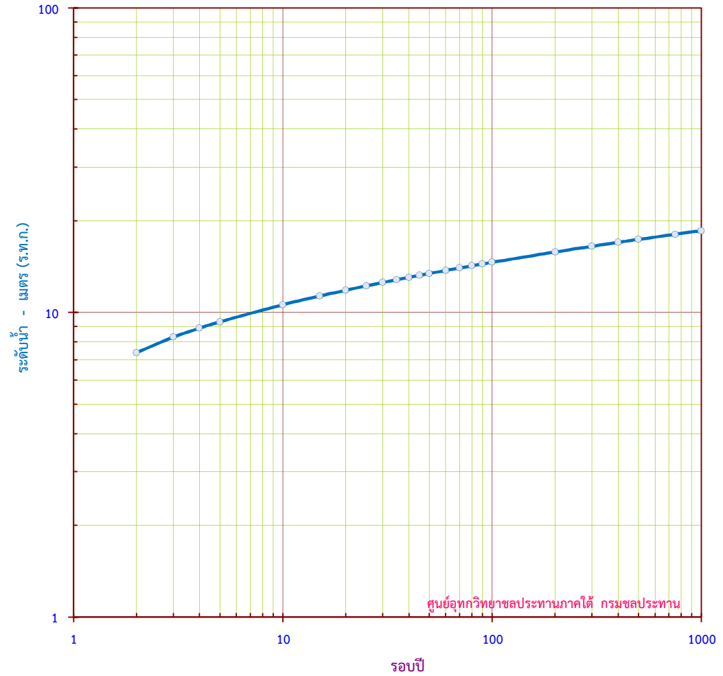
กราฟแสดง ระดับน้ำสูงสุดรายปี ขนาดรอบปีต่างๆ สถานี X.174 บ.คลองหะ อ.หาดใหญ่ จ.สงขลา
