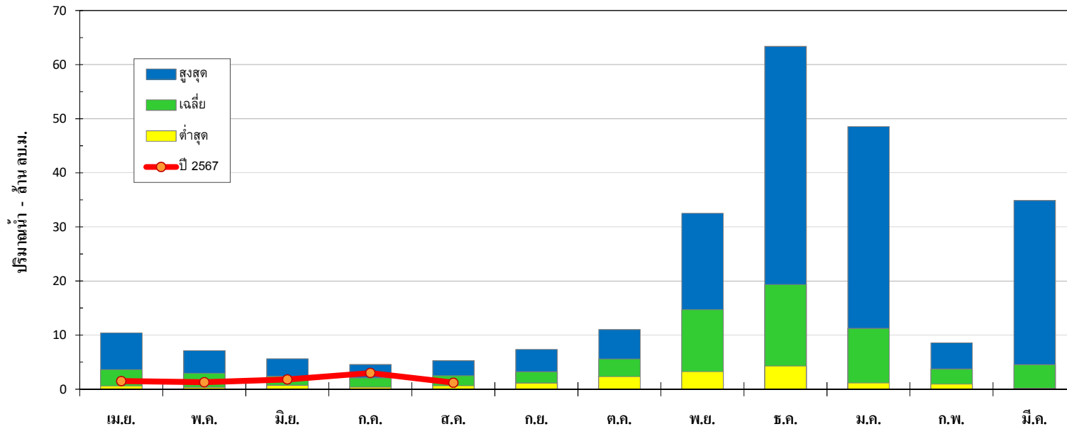
กราฟปริมาณน้ำท่ารายเดือน คลองท่ามะ(บน) ปีน้ำ 2552-2566 สถานี X.276 บ.เขาปู่ อ.ศรีบรรพต จ.พัทลุง
