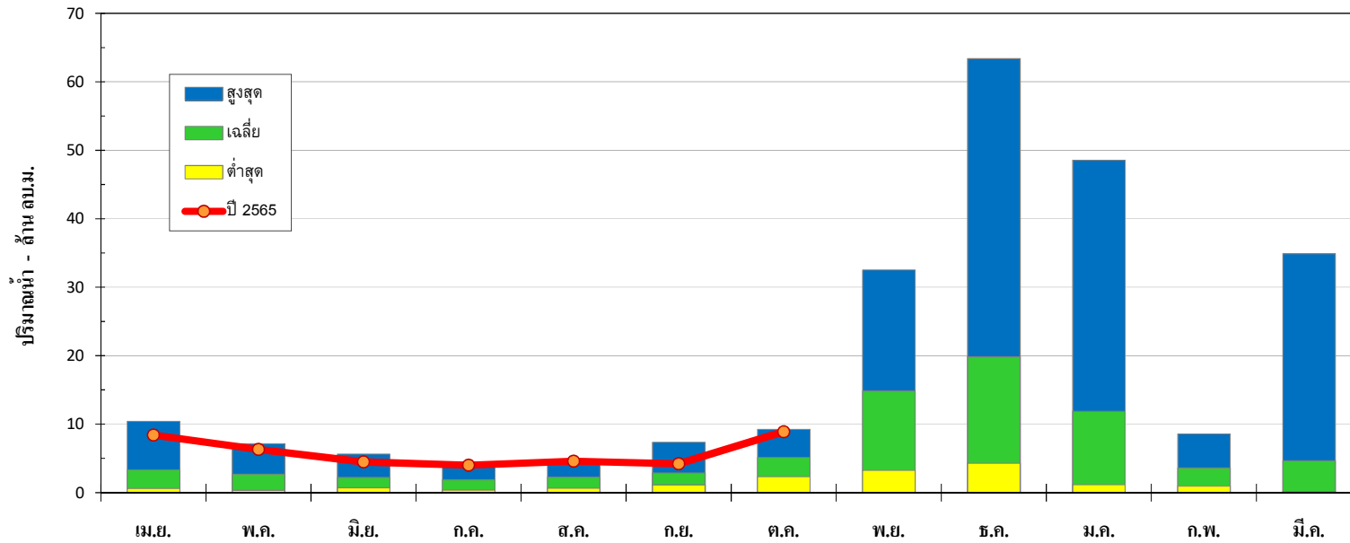
กราฟปริมาณน้ำท่ารายเดือน คลองท่ามะ(บน) ปีน้ำ 2552-2564 สถานี X.276 บ.เขาปู่ อ.ศรีบรรพต จ.พัทลุง
